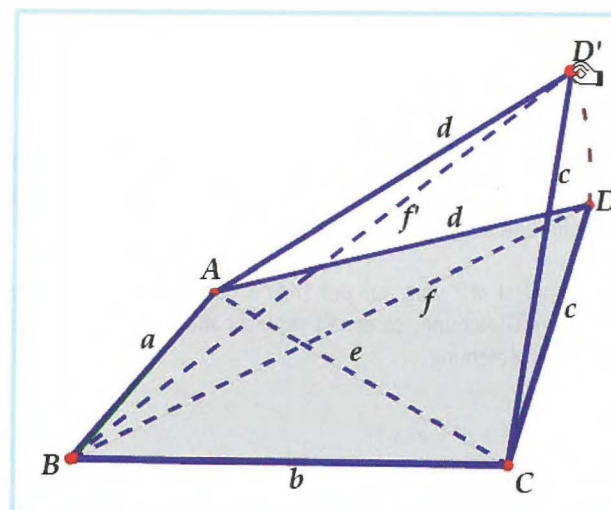
Abb. 1. Auffaltung eines ebenen Vierecks
