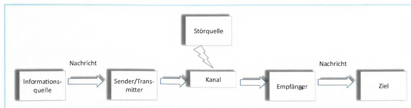
Abb. 1. Kommunikationsmodell nach SHANNON in Anlehnung an MARTIGNON (2015)
