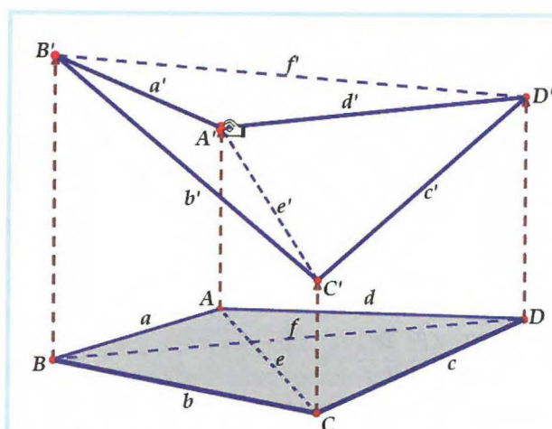
Abb. 2. Verräumlichung durch Erhebung von Eckpunkten
