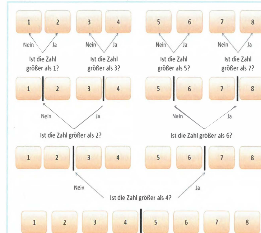
Abb. 4. Fragenbaum zur »Obere Hälfte«-Strategie
