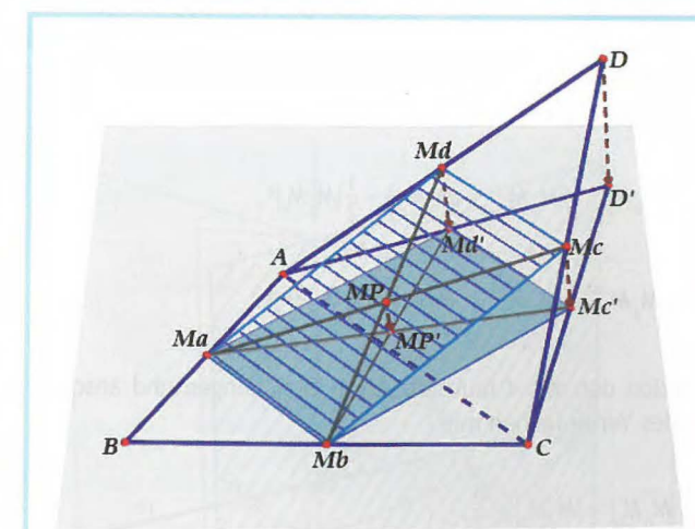
Abb. 3. Beweisfigur zu Aussage (1)
